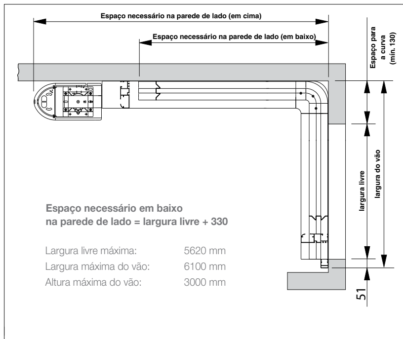
Medidas de montagem (visto de cima)
